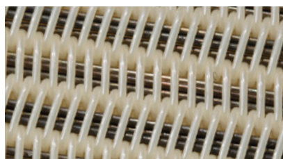
Gefüllte PPS-Spiralsiebe
