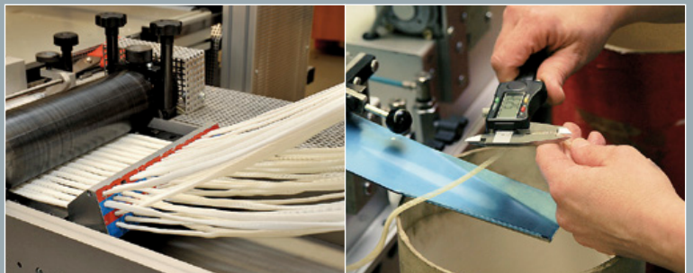
Fügen von Spiralsieben
